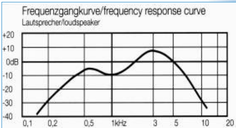
Frequenzgang Lautsprecher
