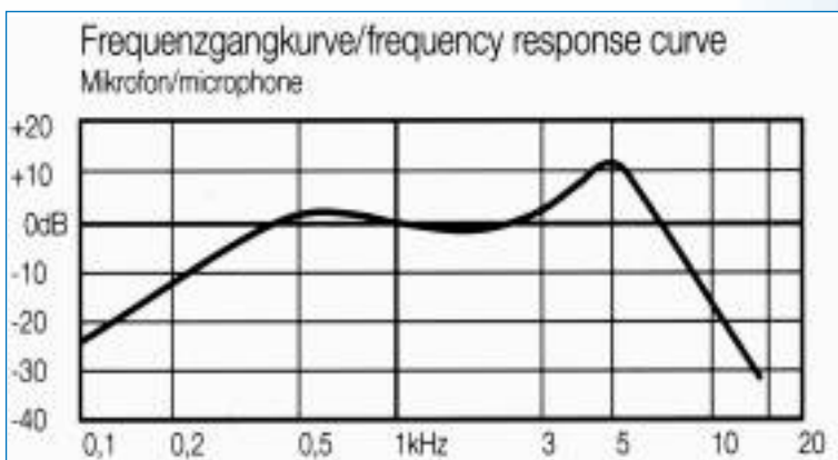
Frequenzgang Mikrofon
